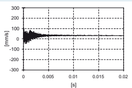
Nachschwingung AllGrip
