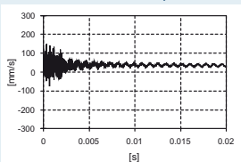
Nachschwingung Standard-Schrumpffutter
