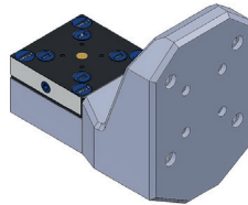
44090-SO000113 L-Winkel
