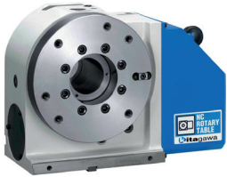
MR200 (Abb. zeigt Version mit Motor rechts)
